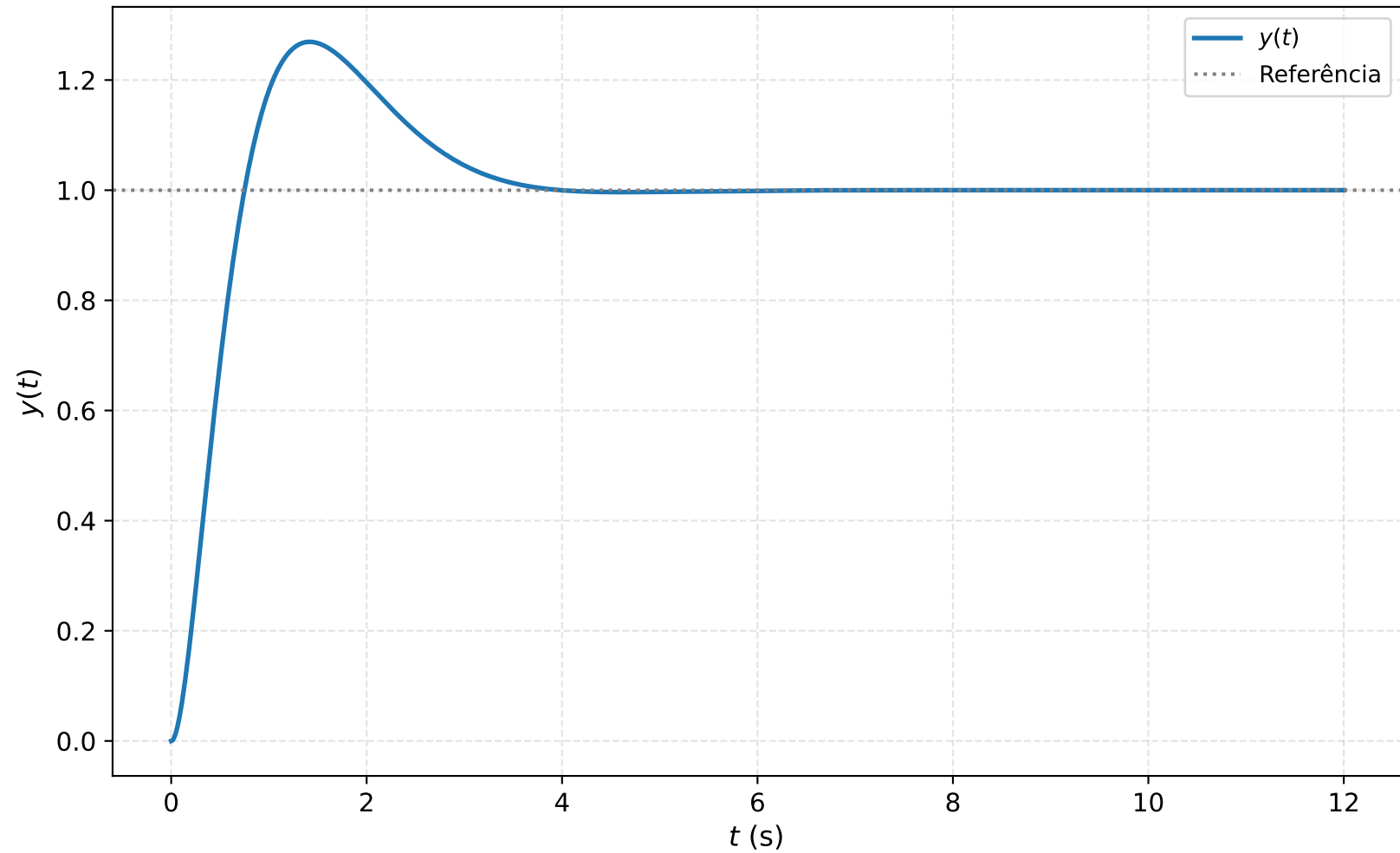
Resposta ao degrau unitário — malha fechada
